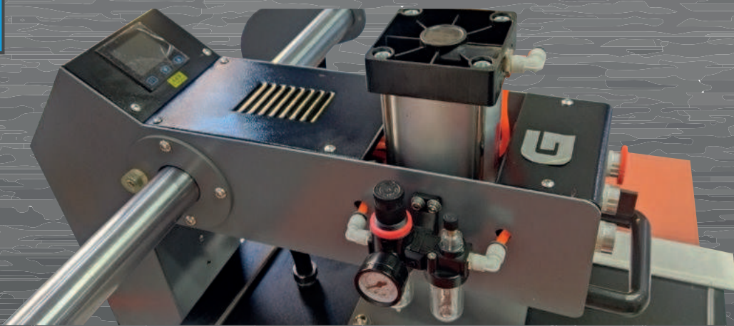
CONEXION NEUMATICA
